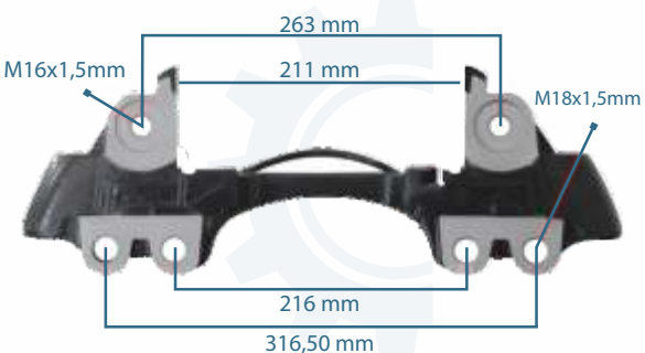
133216 CALIPER CARRIER 22.5 PAN22 RIGHT 3 080 007221 - 3 080 007420 - 640 195 069 0 - 640 195 075 0
