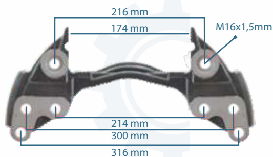
111331 CALIPER CARRIER MB ATEGO K000358 - 000 421 1606
