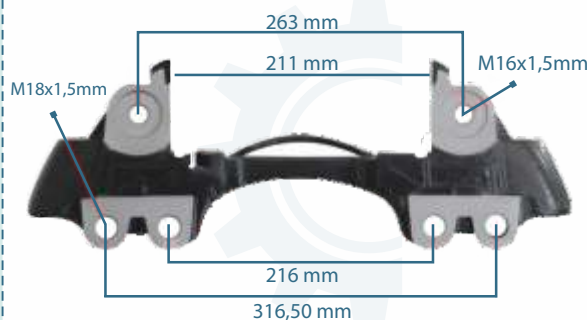
133215 CALIPER CARRIER 22.5 PAN22 LEFT 3 080 007121 - 3 080 007320 - 640 195 068 0 - 640 195 074 0
