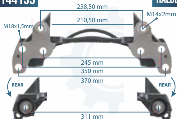
144135 CALIPER CARRIER MODUL X
